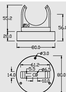
Art. MGP01/OBO01 Magnete con collare in PVC per lampada Ø 50 mm
