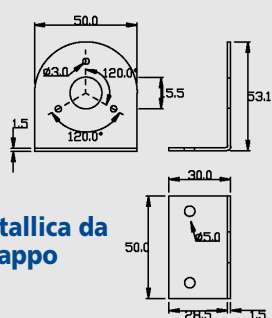
(Staffa metallica da fissare al tappo lampada Ø 40/43 mm)
