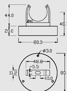
Art. MGP01/OBO02 Magnete con collare in PVC per lampada Ø 40/43 mm
